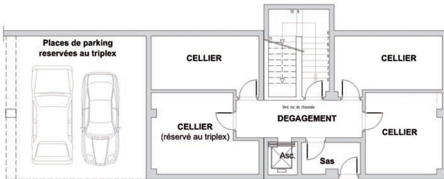
Plan SOUS-SOL
